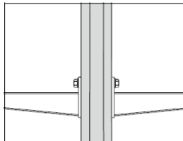
Montage van een console 50 d.m.v. een T-bout.
