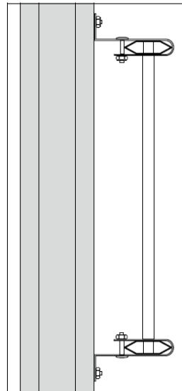
Een kabelladder kan verticaal of horizontaal op een pendelprofiel 24/20FS gemonteerd worden d.m.v. een wandbeugel 11/25 of 11/75 en T-bouten.
