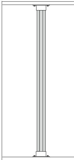
Een pendelprofiel 24/20FS kan als staander tussen vloer en plafond gemonteerd worden d.m.v. 2 profielsteunen 24/20FS.
