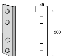
Eclisse d'assemblage 2FJ
