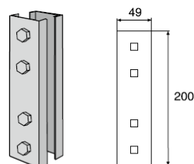
Eclisse d'assemblage 20J
