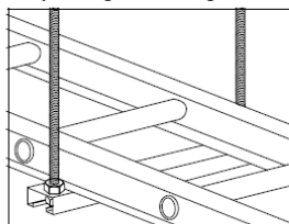
Draagconsole HSO M10 gemonteerd met draadstang M10.
