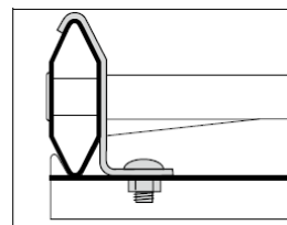
Met profielklem 42 maakt u de kabelladder vast aan de draagconsole HSO.
