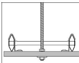
Centrale ophanging met draagconsole HSO M16, breedtes 400-600, draadstang M16, 2 moeren M16 en onderlegplaat HSO M16.
