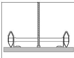
Centrale ophanging met draagconsole HSO M10, breedtes 150-300, draadstang M10 W76 en 2 moeren M10.
