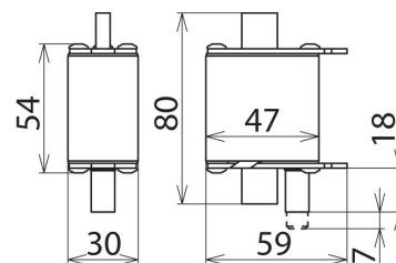
Dimensions VA NH00 280 FM
