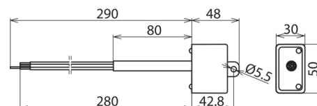
Dimensions DCOR L 3P 275 SO IP
