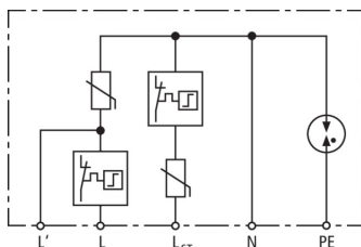
Schéma de principe du circuit DCOR L 3P 275 SO IP
