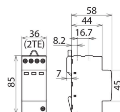
Dimensions DG TT 2P 5 275 NL
