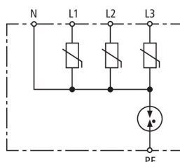
Schéma de principe du circuit DG TT 5 275 NL
