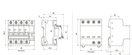
Dimension drawing SPD+POP+MCB 32A 3P+N T1+2
