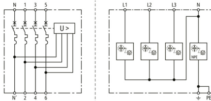
Basic circuit diagram SPD+POP+MCB 40A 3P+N T1+2
