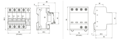
Dimension drawing SPD+POP+MCB 40A 3P+N T1+2
