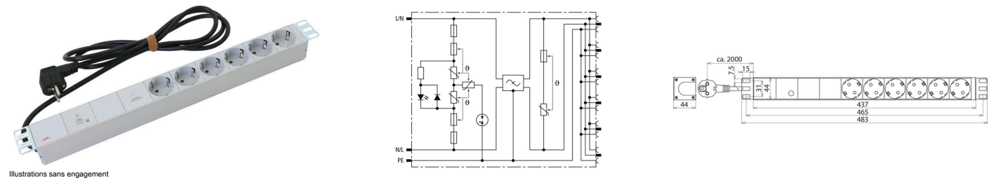
Réglette avec protection antisurtension et filtre réseau pour baie 19 pouces. Schéma de principe du circuit SFL PRO 6X 19" Dimensions SFL PRO 6X 19"
