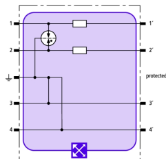
Schéma de principe du circuit BXT ML2 B 180
