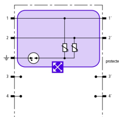
Schéma de principe du circuit BXT ML2 MY 250
