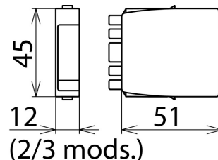
Dimensions BXT ML4 BD 48
