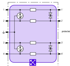
Schéma de principe du circuit BXT ML4 BD 48
