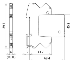
Dimension du BCO ML2 BE HF 5
