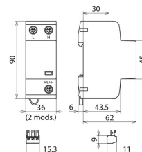
Dimensions DSH B TT 2P 255 FM
