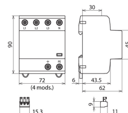
Dimensions DSH B TT 255 FM
