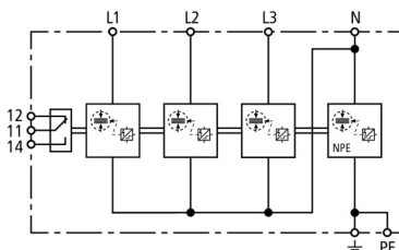
Schéma de principe du circuit DSH B TT 255 FM
