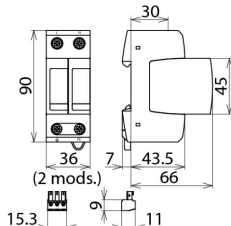
Dimensions DG MP TT 2P 275
