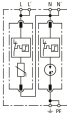
Schéma de principe du circuit DG MP TT 2P 275
