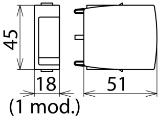
Dimensions DGP C MOD
