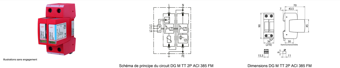
Parafoudre modulaire avec Interrupteur de Circuit Avancé (ACI) pour les systèmes monophasés 230 V TT et TN (circuit 1 + 1).
