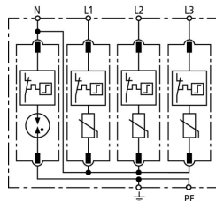
Schéma de principe du circuit DG M TT 275 NL
