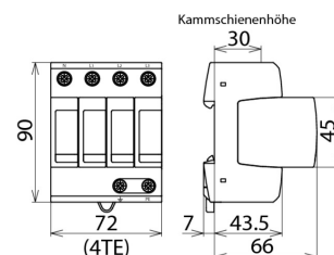
Dimensions DG M TT 275 NL
