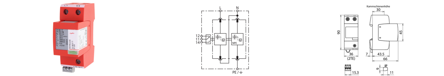
Schéma de principe du circuit DV M2 TT 2P 255 FM Dimensions DV M2 TT 2P 255 FM Parafoudre combiné modulaire pour systèmes TT et TN (mode de connexion 1 + 1).
