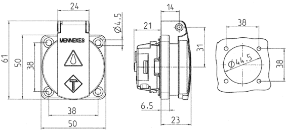
Schéma 1 MB 410 Dim. en mm
